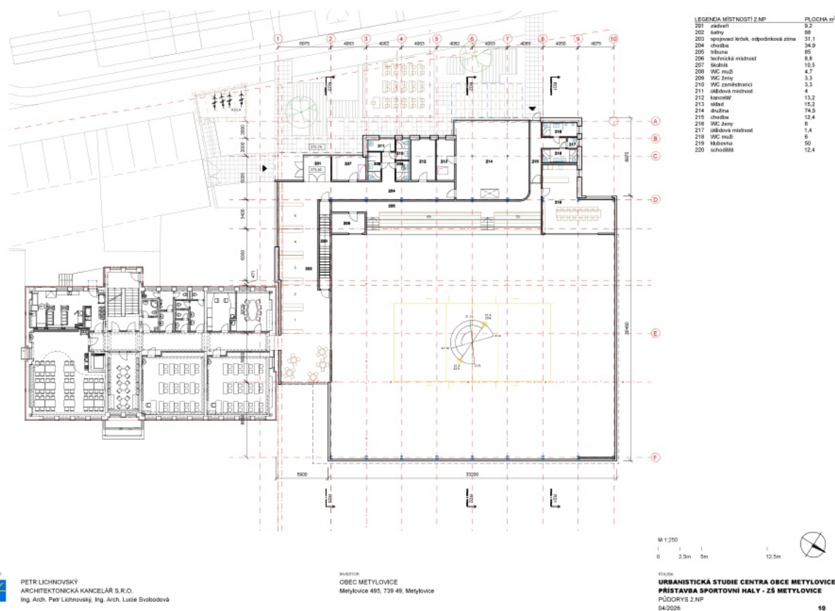
Půdorys 2.NP
