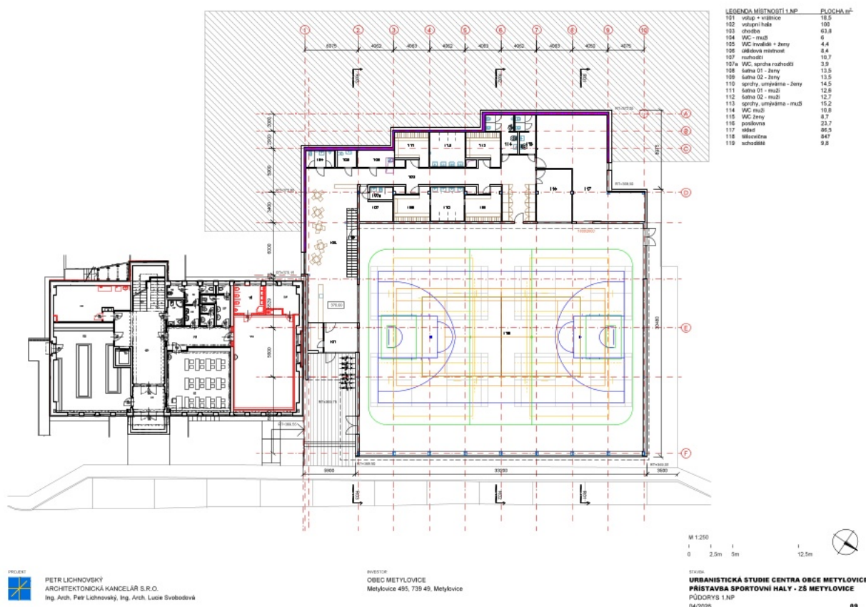
Půdorys 1.NP
